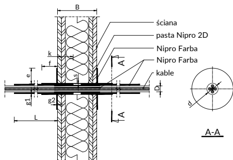
Rys. Zabezpieczenie przejść pojedynczego kabla lub wiązki kabli przez ścianę wykonane przy użyciu Nipro Farby i Pasty 2D.
